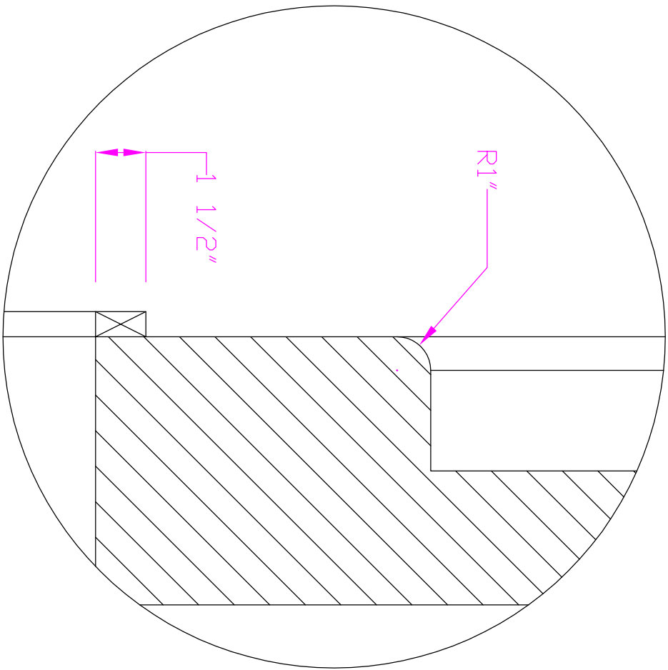
B D15 MOLDING SECTION
