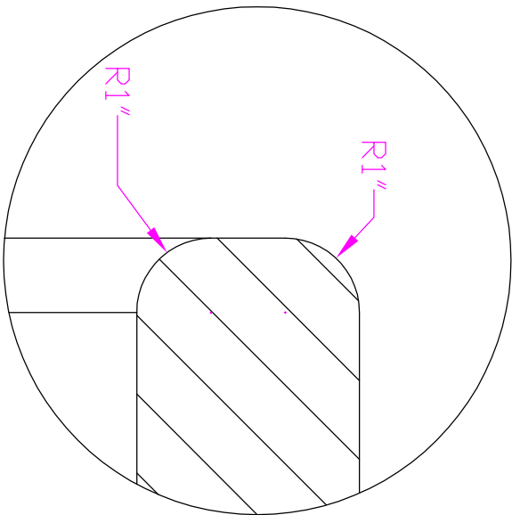
C D15 MOLDING SECTION
