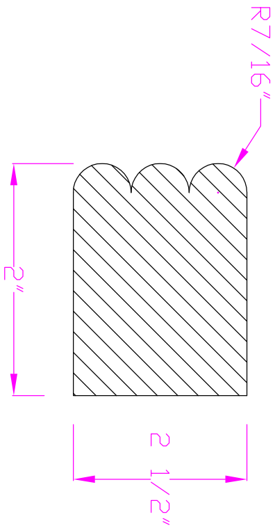
F D15 MOLDING SECTION
